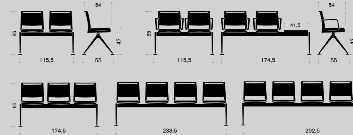
Beam seating Bancada Poutre
