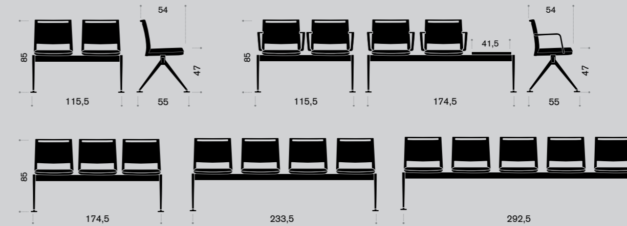
Beam seating Bancada Poutre
