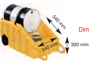
Ref. 3065 carro volteador de bidones
