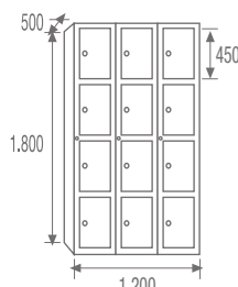
STV4-40/3 COD. 44043
