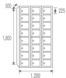
STV8-40/3 COD. 44083
