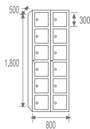
STV6-40/2 COD. 44062
