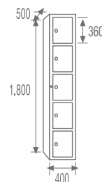
STV5-40/1 COD. 44051
