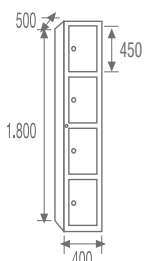
STV4-40/1 COD. 44041
