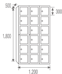
STV6-40/3 COD. 44063
