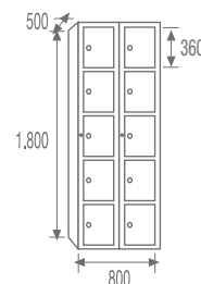
STV5-40/2 COD. 44052
