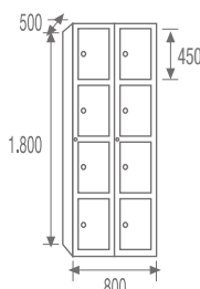
STV4-40/2 COD. 44022
