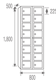
STV8-40/2 COD. 44082
