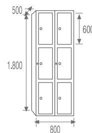
STV3-40/2 COD. 44032
