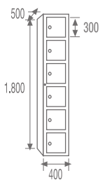
STV6-40/1 COD. 44061
