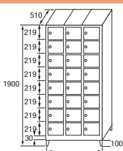
SZ-30/3 COD. 43083
