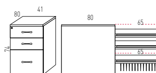
CAJÓN + ARCHIVO CARPETERO CON BASTIDOR
